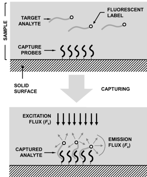
Σχήμα 5: Αρχή λειτουργίας του ανιχνευτή DNA
