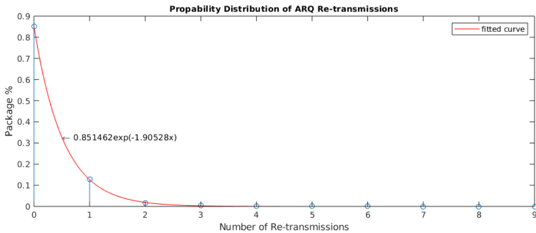
Σχήμα 3: Διάγραμμα κατανομής του αριθμού εκπομπών ανά πακέτο, για σύνοδο ARQ 60 λεπτών, καθώς και εκτίμηση της κατανομής της πιθανότητας σφάλματος.
