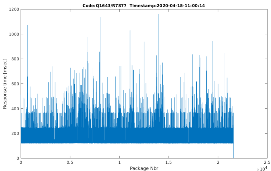
Σχήμα 2: Διάγραμμα απόκρισης του συστήματος για κάθε επιτυχή αποστολή ARG 60 λεπτών
