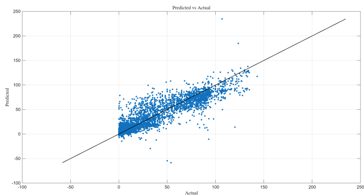
Σχήμα 14: Σύγκριση Predicted vs Actual στο test set.
