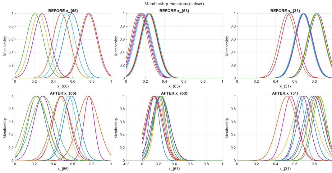
Σχήμα 16: Ενδεικτικές MF για επιλεγμένες εισόδους πριν/μετά την εκπαίδευση.
