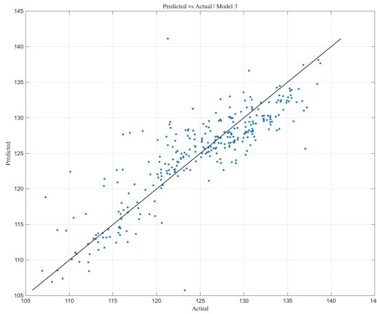
(α') Predicted vs Actual — Model 3
