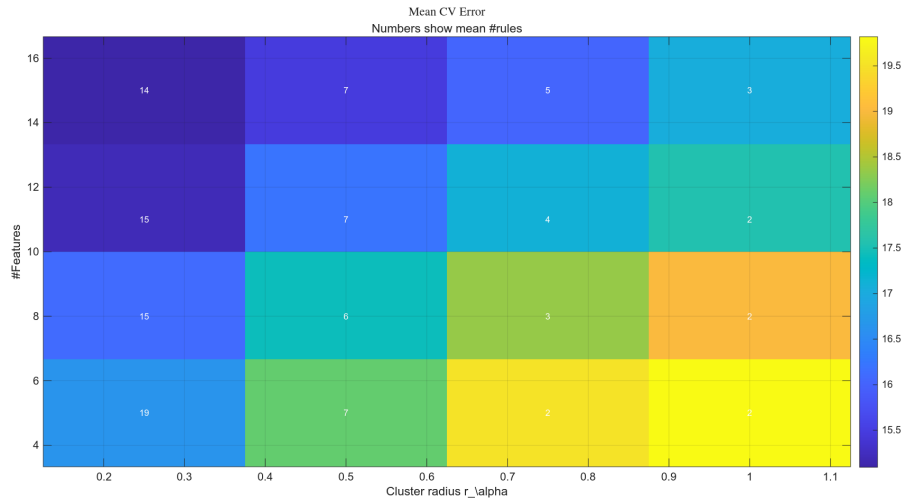
Σχήμα 11: Heatmap μέσων σφάλματος CV ανά (k_{\text{feat}}, r_{\alpha}) — με επικάλυψη του #κανόνων.
