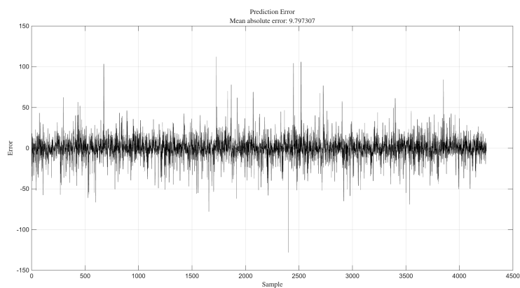
Σχήμα 15: Residuals (σειρά σφάλματος) στο test set.
