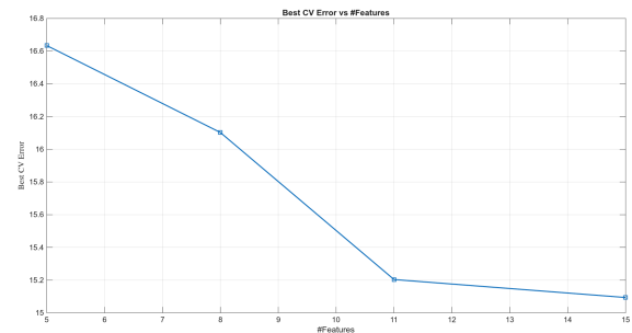
Σχήμα 12: Σχέση σφάλματος με πολυπλοκότητα (κανόνες) και μείωση διαστασιμότητας (χαρακτηριστικά).
