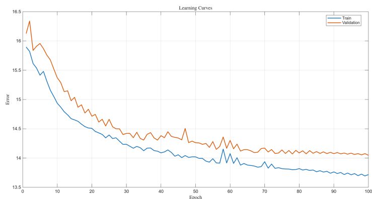
Σχήμα 13: Καμπύλες μάθησης του τελικού μοντέλου (train/validation).
