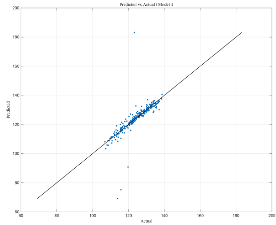
(β') Predicted vs Actual — Model 4
