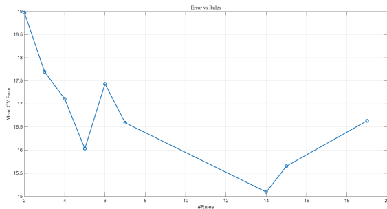
Σχήμα 12: Σχέση σφάλματος με πολυπλοκότητα (κανόνες) και μείωση διαστασιμότητας (χαρακτηριστικά).
